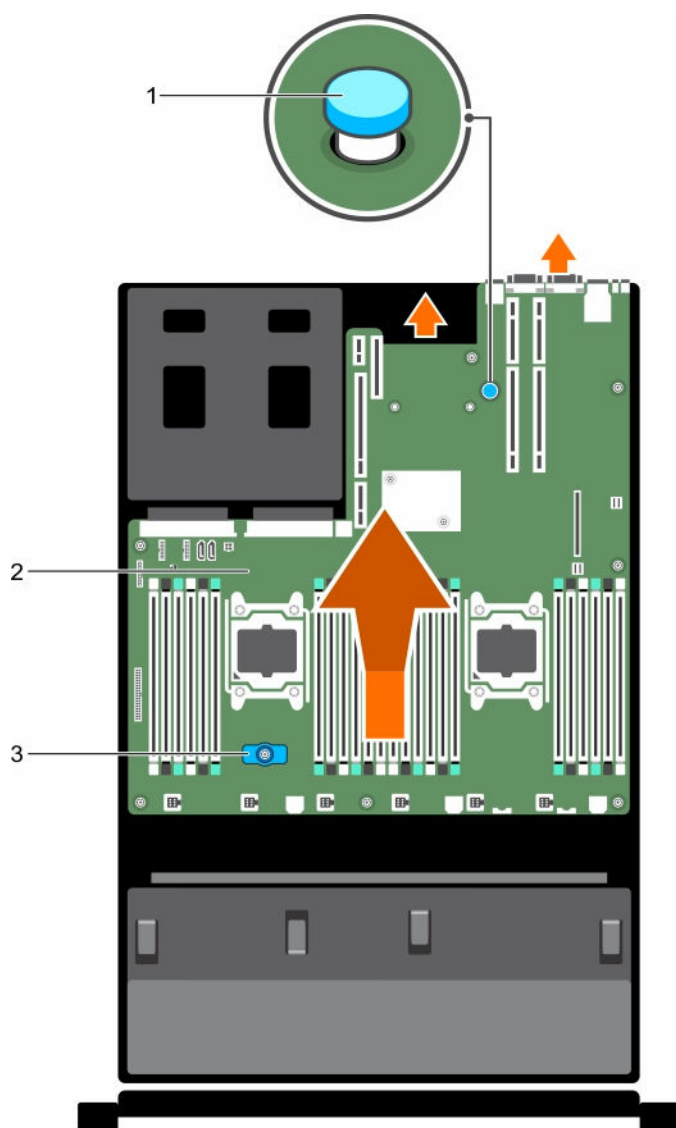
图 63: 安装系统板
