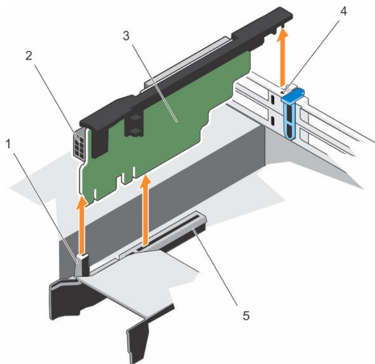
图 43: 卸下扩展卡提升板 3
