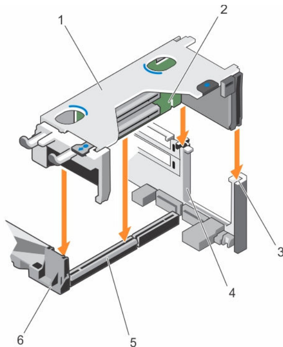
图 46: 安装扩展卡提升板 1
