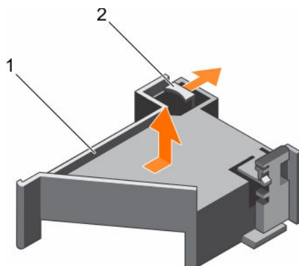
图 25: 卸下 PCIe 卡固定器
