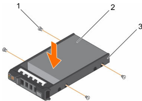
图 72: 将硬盘驱动器安装到硬盘驱动器托盘中
