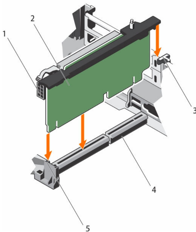
图 47: 安装扩展卡提升板 2
