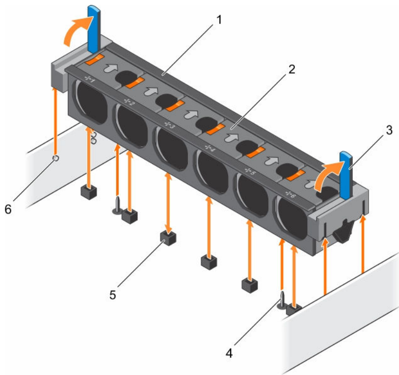
图 15: 卸下冷却风扇部件
