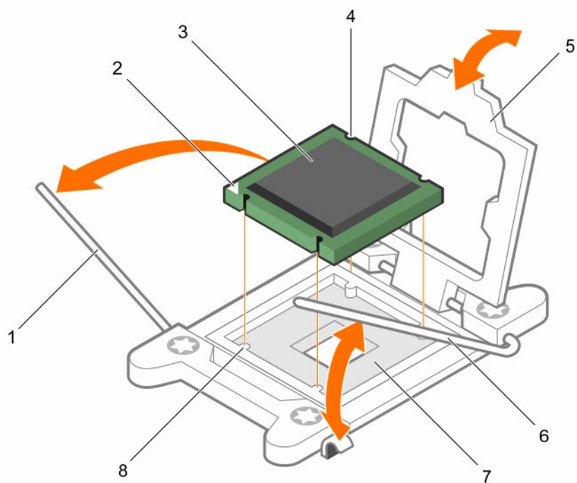
图 22: 卸下处理器
