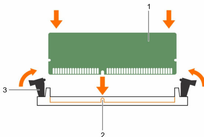
图 19: 安装内存模块
