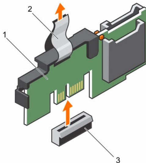
图 51: 卸下内部双 SD 模块 (IDSDM)
