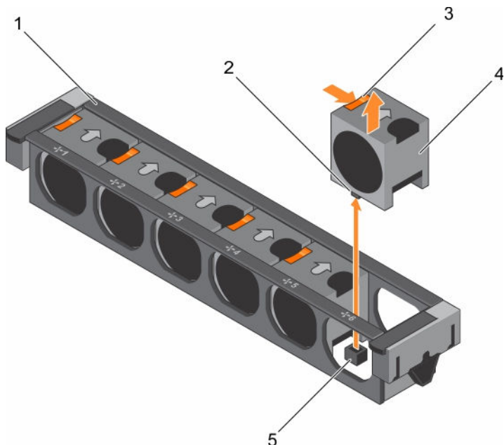
图 14: 卸下冷却风扇
