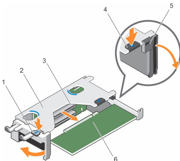
图 35: 从扩展卡提升板 1 上卸下扩展卡
