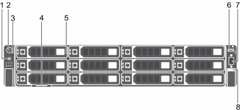
图 1: Dell DR6300 系统前面板功能部件和指示灯
