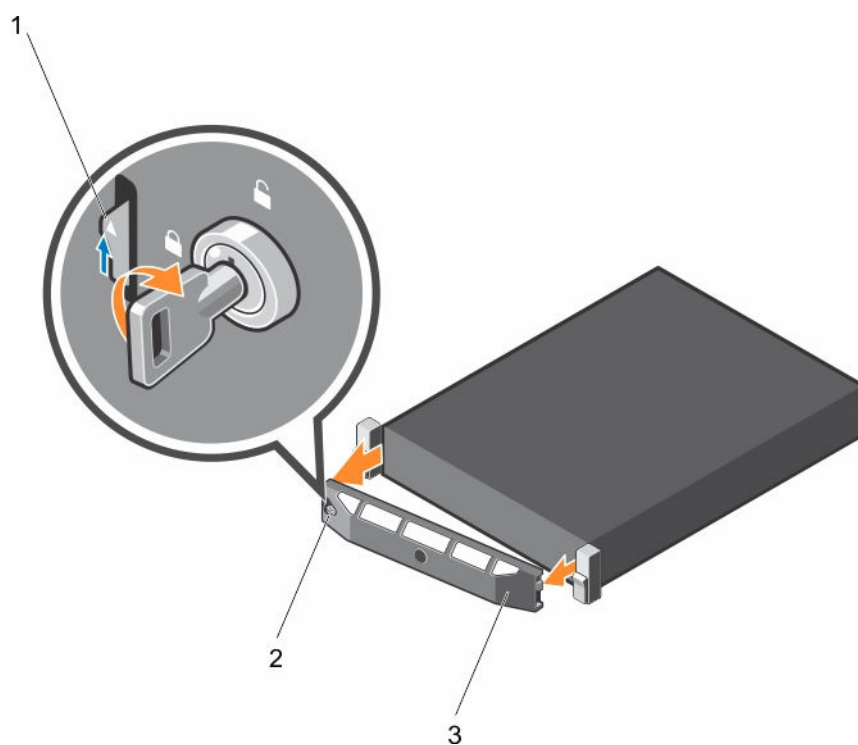
图 9: 卸下可选的前挡板
