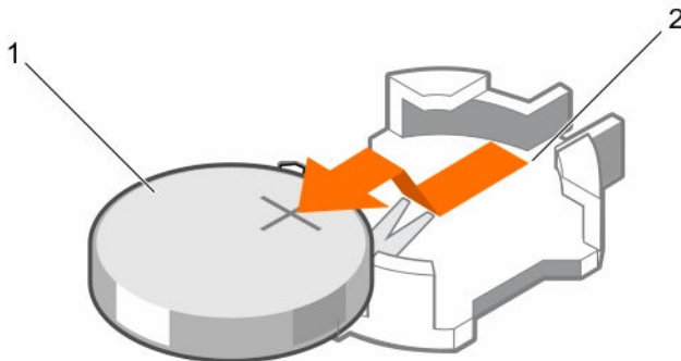
图 56: 卸下系统电池
