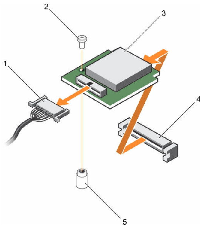
图 80: 卸下 vFlash 介质单元
