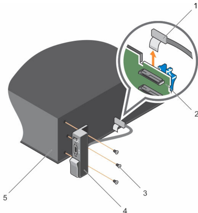
图 84: 卸下 I/O 面板
