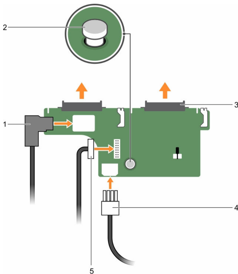
图 77: 安装可选的 2.5 英寸 (x2) 硬盘驱动器背板
