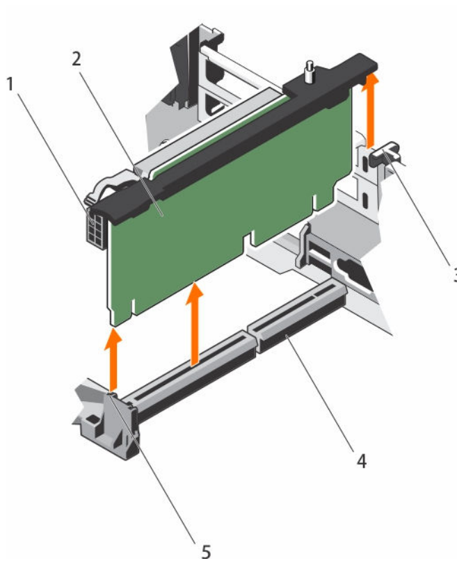
图 41: 卸下扩展卡提升板 2
