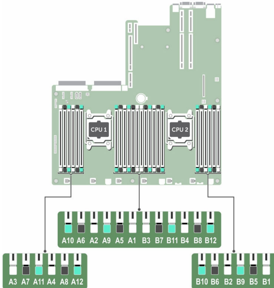
图 17: 内存插槽位置
