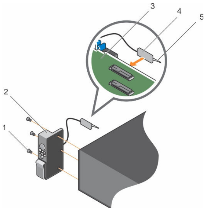
图 83: 安装控制面板
