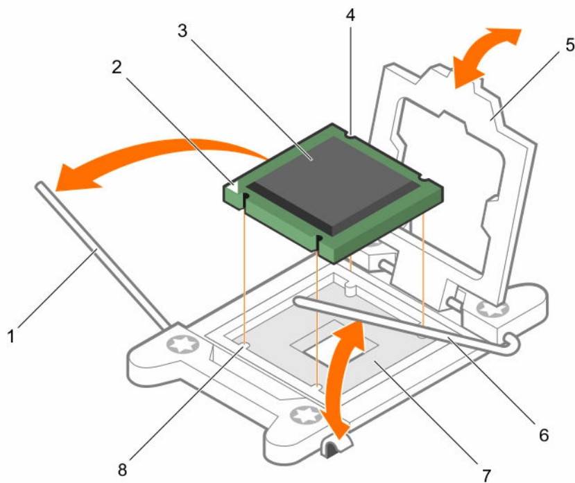
图 23: 安装处理器
