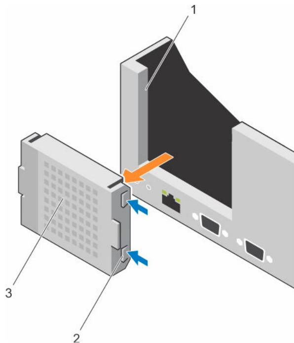
图 37: 卸下提升板 1 挡片
