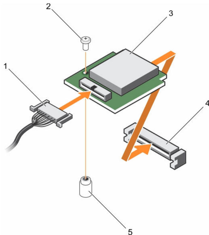
图 81: 安装 vFlash 介质单元
