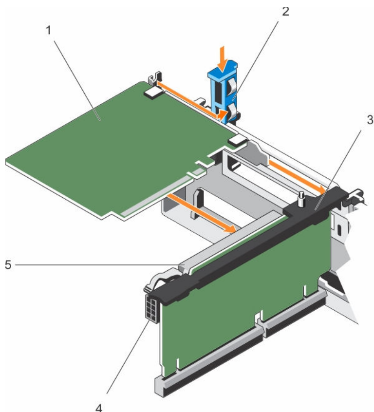
图 34: 将扩展卡安装到扩展卡提升板 2 或 3 中
