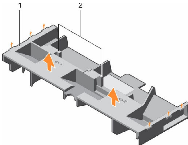
图 13: 卸下冷却导流罩
