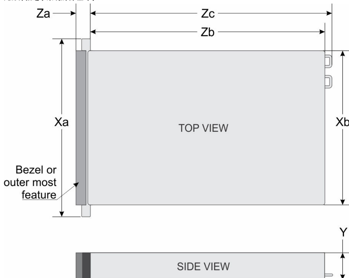
图 8: Dell DR6300 系统的机箱尺寸
