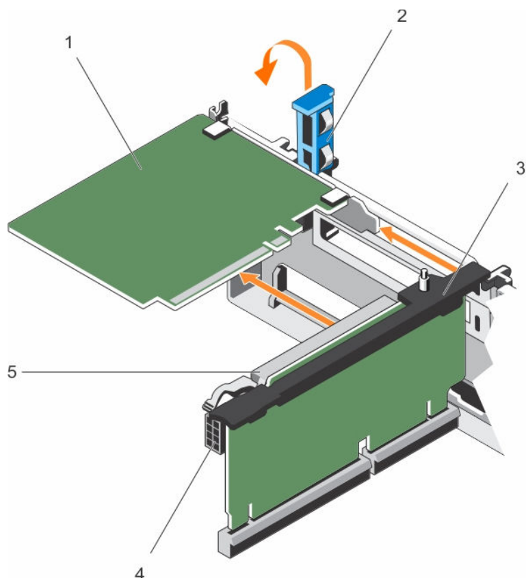
图 33: 从扩展卡提升板 2 或 3 中卸下扩展卡
