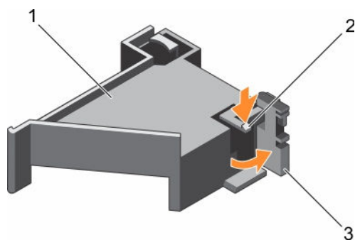
图 27: 打开 PCIe 卡固定器门锁
