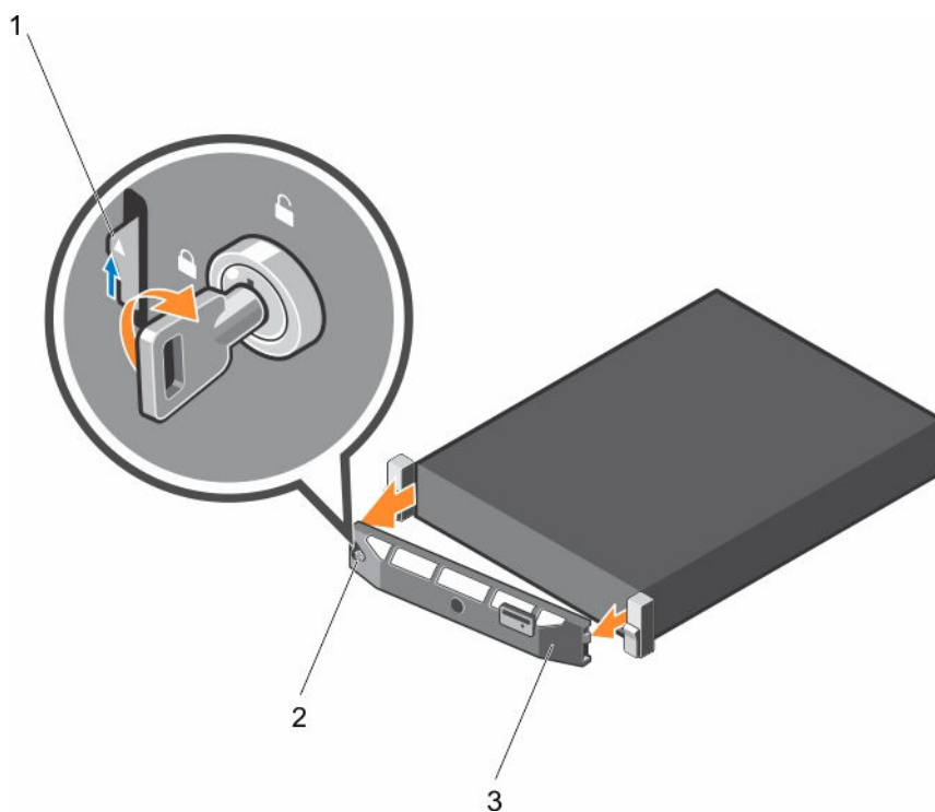
图 10: 卸下可选的快速同步前挡板
