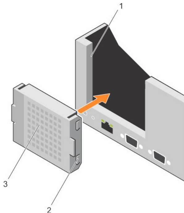
图 38: 安装提升板 1 挡片
