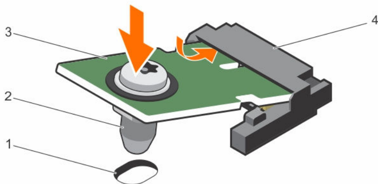
图 64: 安装 TPM
