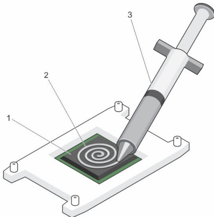
图 24: 在处理器顶部涂抹导热油脂
