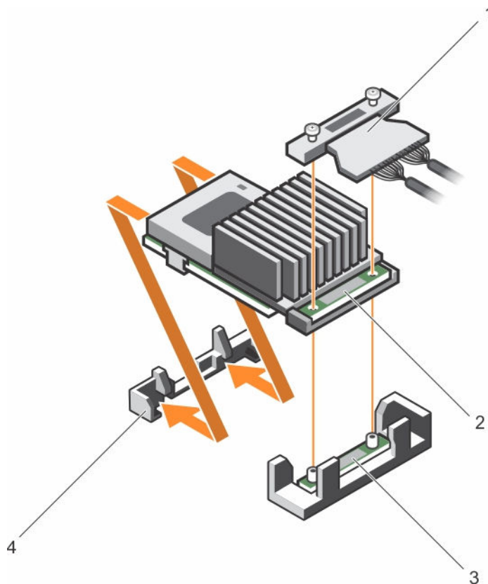
图 32: 安装集成存储控制器卡
