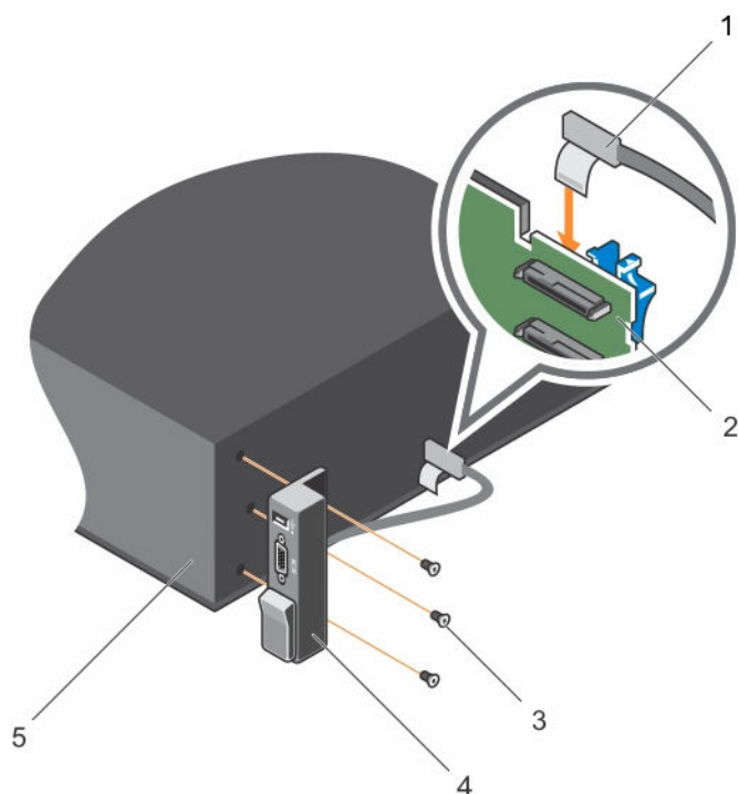
图 85: 安装 I/O 面板
