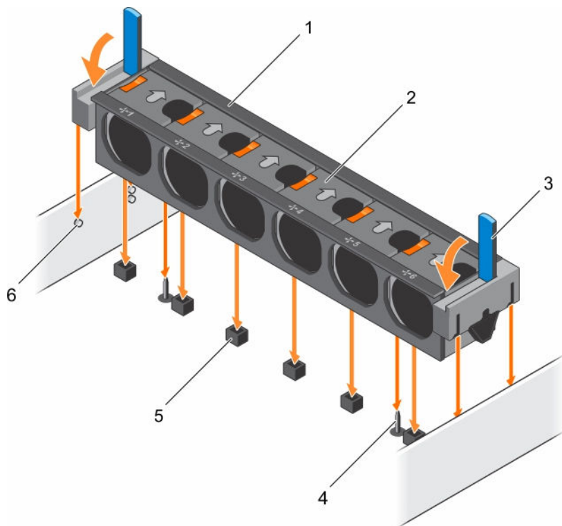
图 16: 安装冷却风扇部件
