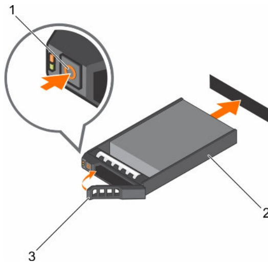
图 70: 安装热插拔硬盘驱动器或 SSD
