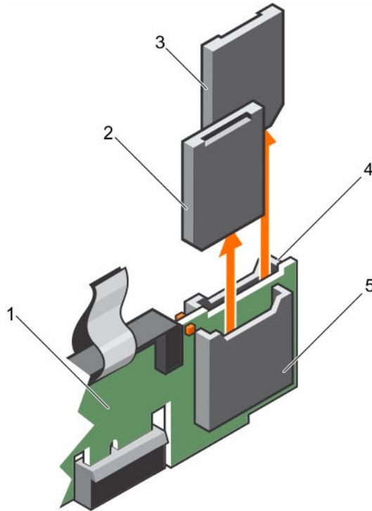
图 49: 卸下内部 SD 卡
