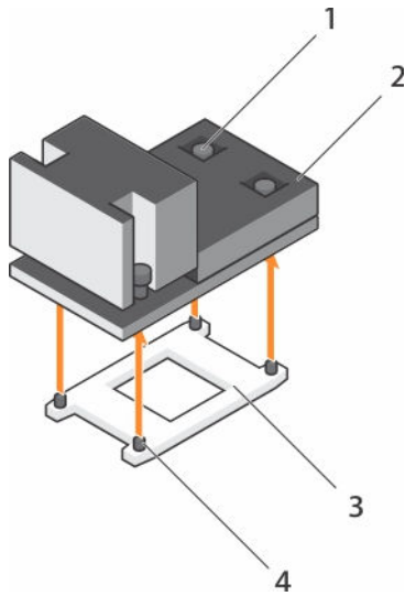
图 20: 卸下散热器
