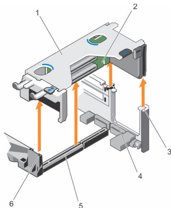
图 39: 卸下扩展卡提升板 1
