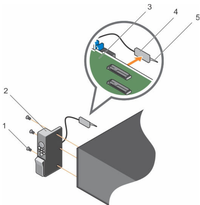
图 82: 卸下控制面板
