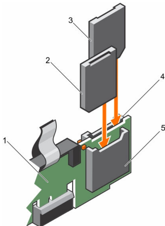
图 50: 安装内部 SD 卡
