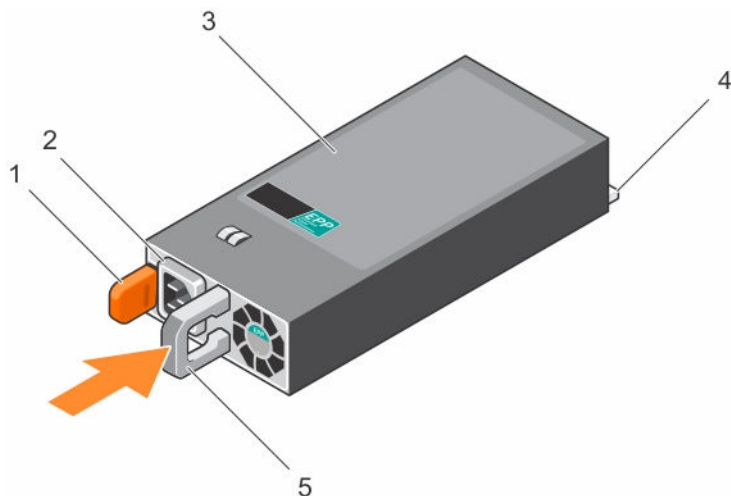
图 61: 安装交流 PSU
