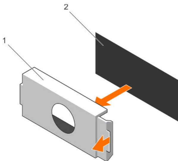
图 58: 卸下 PSU 挡片
