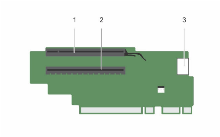
图 44: 识别扩展卡提升板 3 上的连接器（默认）
