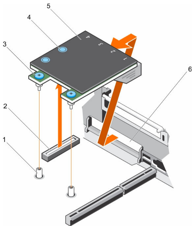
图 52: 卸下 NDC
