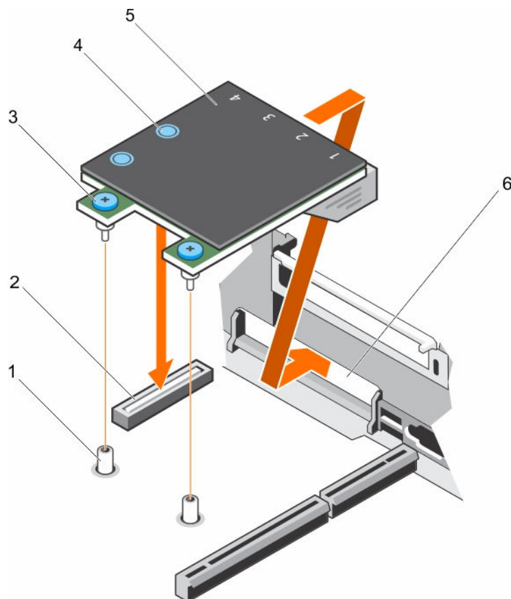
图 53: 安装 NDC
