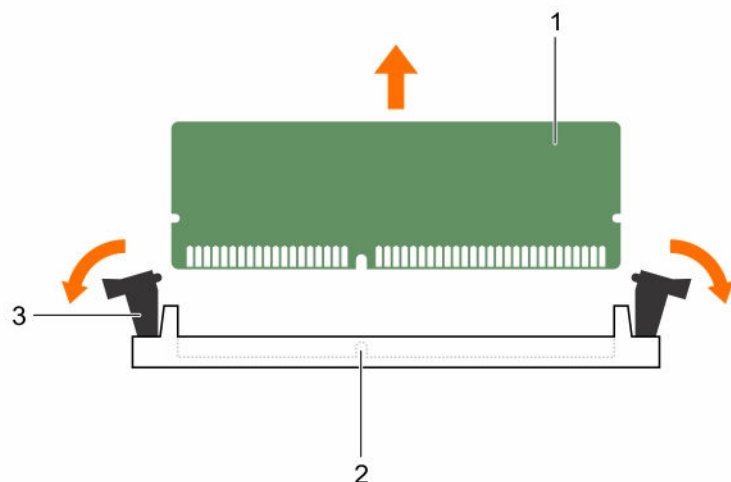
图 18: 卸下内存模块
