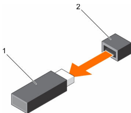
图 54: 卸下内置 USB 存储盘
