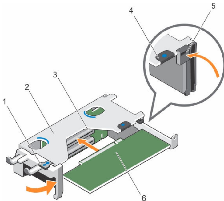
图 36: 将扩展卡安装到扩展卡提升板 1 中
