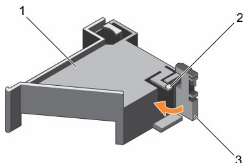
图 28: 关闭 PCIe 卡固定器门锁
