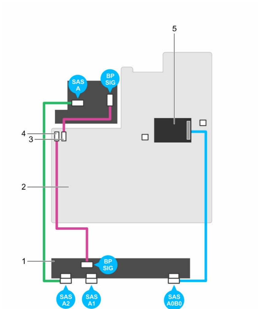
图 74: 布线图 — 3.5 英寸 (x12) SAS/SATA 背板
