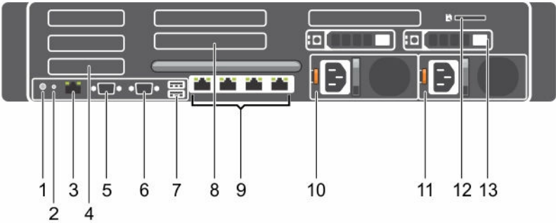
图 2: 背面板功能部件
