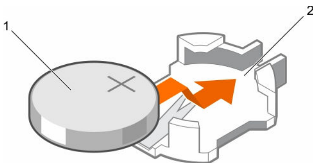
图 57: 安装系统电池
