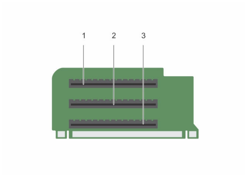
图 40: 识别扩展卡提升板 1 上的连接器
