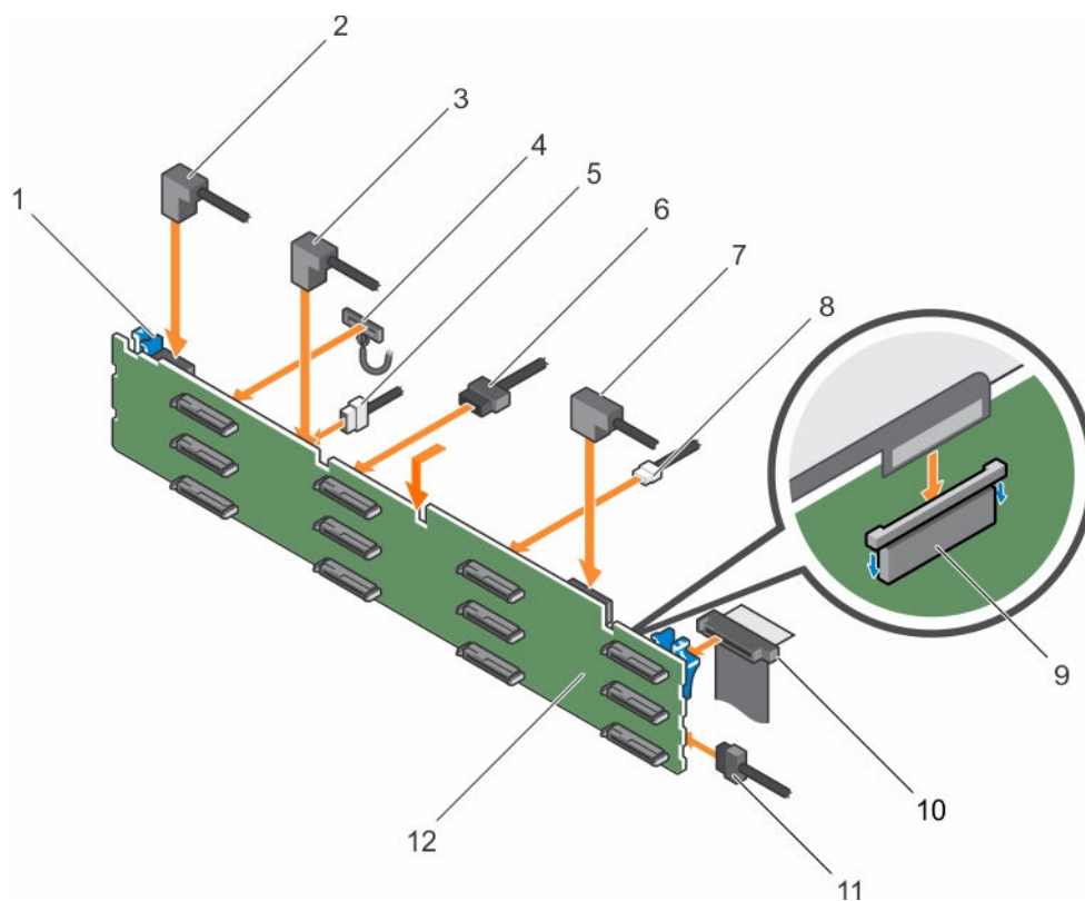
图 75: 安装 3.5 英寸 (x12) SAS/SATA 背板
