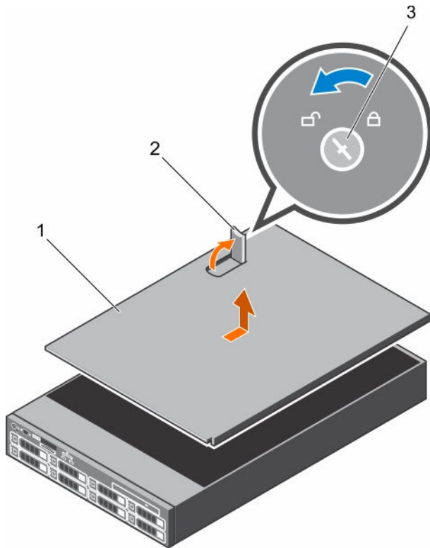
图 11: 卸下系统护盖
