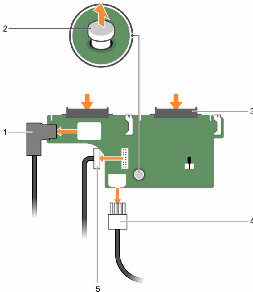
图 76: 卸下可选的 2.5 英寸 (x2) 硬盘驱动器背板
