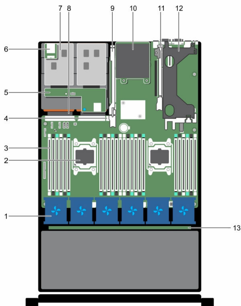
图 12: 系统内部
