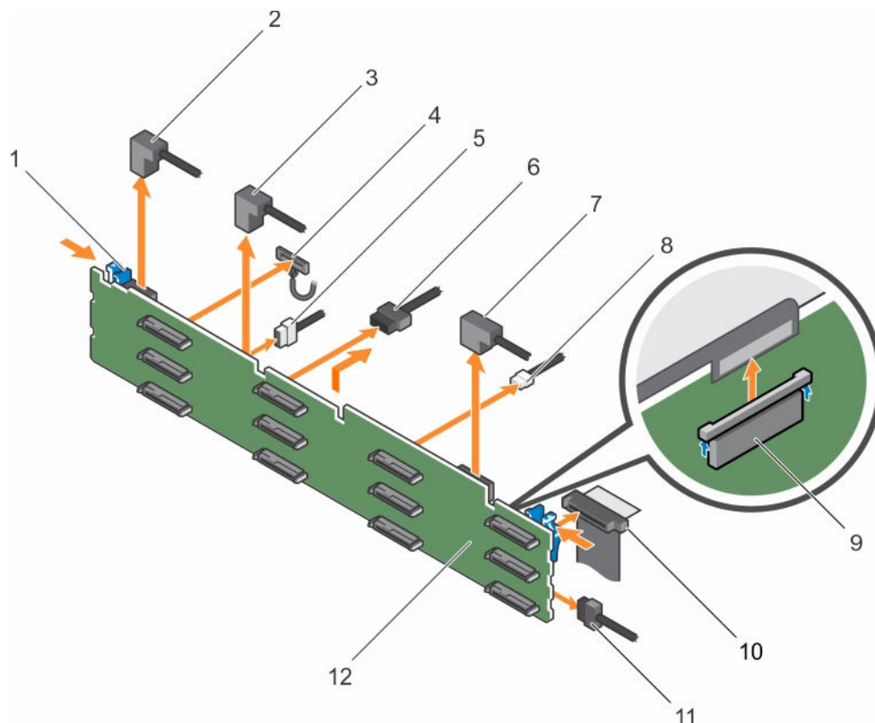
图 73: 卸下 3.5 英寸 (x12) SAS/SATA 背板
