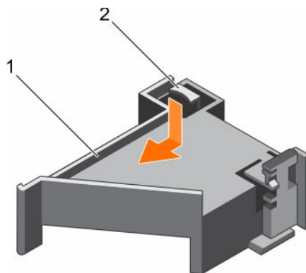
图 26: 安装 PCIe 卡固定器
