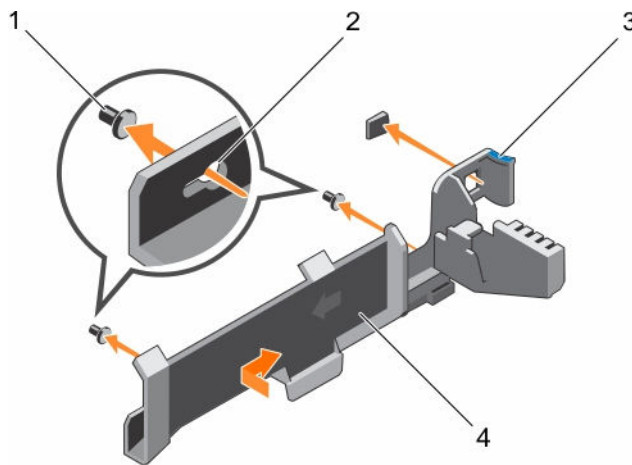
图 30: 安装电缆固定支架
