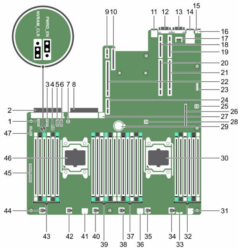
图 86: 系统板跳线和连接器
